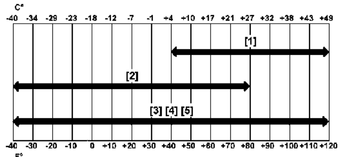
Рис. 255 РЕКОМЕНДУЕМЫЙ КЛАСС ВЯЗКОСТИ ПО ISO (VG) И ИНДЕКС ВЯЗКОСТИ (VI) МАСЛА ГИДРАВЛИЧЕСКОЙ/ГИДРОСТАТИЧЕСКОЙ СИСТЕМЫ
